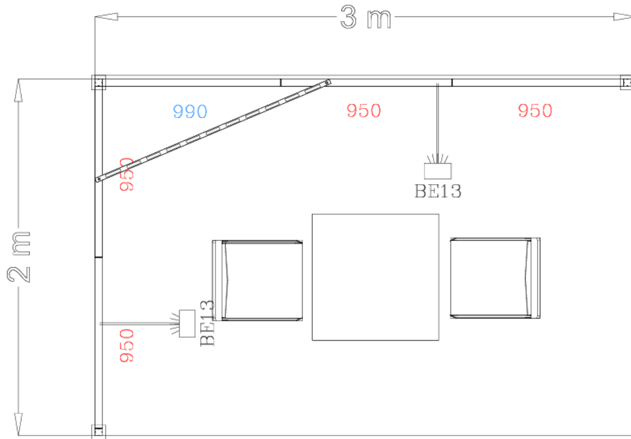
Draufsicht/Top View
