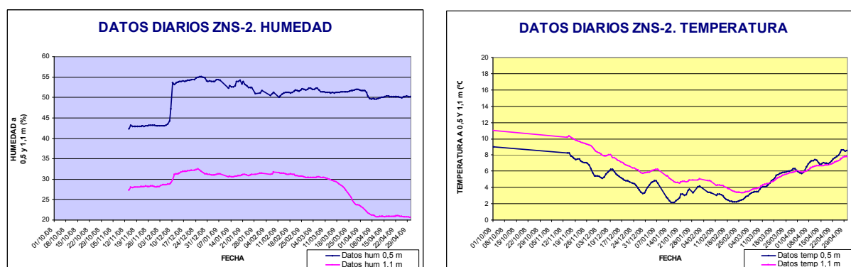
Figuras 6 a) y b). Gráficas de humedad y temperatura registradas en la estación DINA-MAR ZNS 2 de Coca para la duración del 7º ciclo de recarga artificial en la Cubeta de Santiuste. Profundidad de los sensores: 0,5 y 1,1 m.
