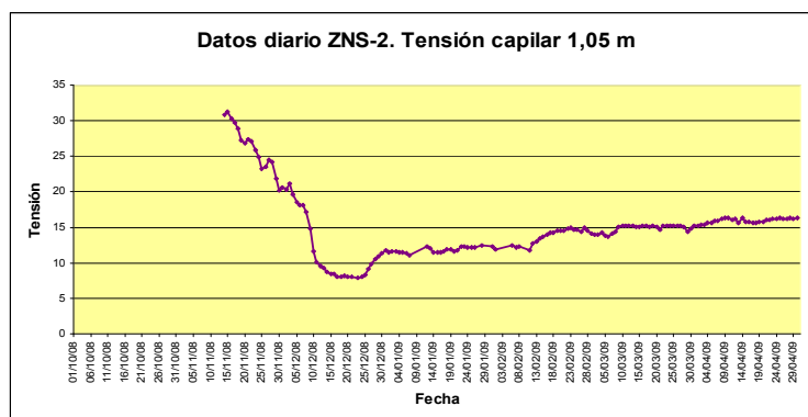
Figura 7. Gráfica de tensión capilar registrada en la estación DINA-MAR ZNS 2. Profundidad del sensor 1,05 m.
