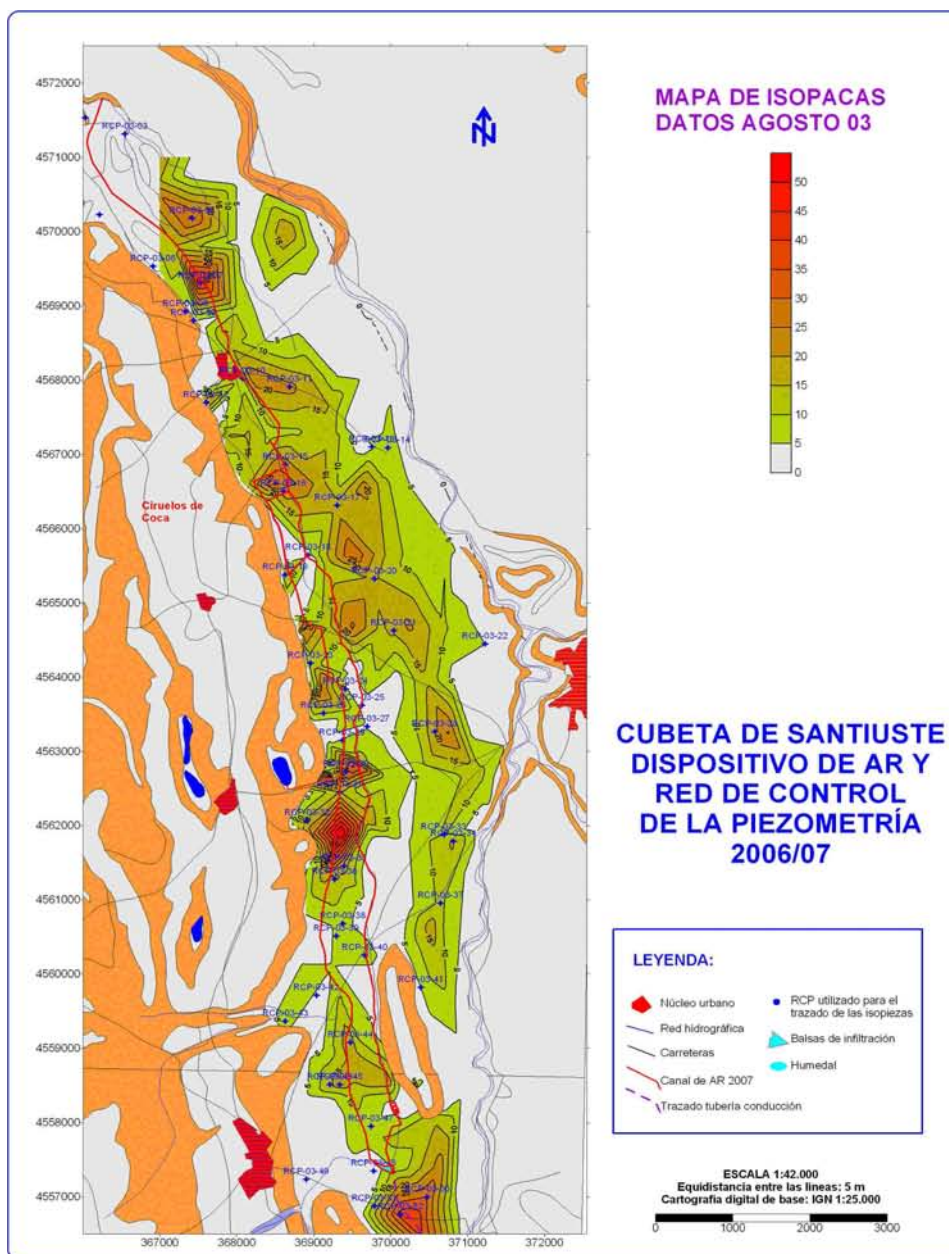
Figura 1. Trazado del dispositivo de recarga artificial de la Cubeta de Santiuste.
