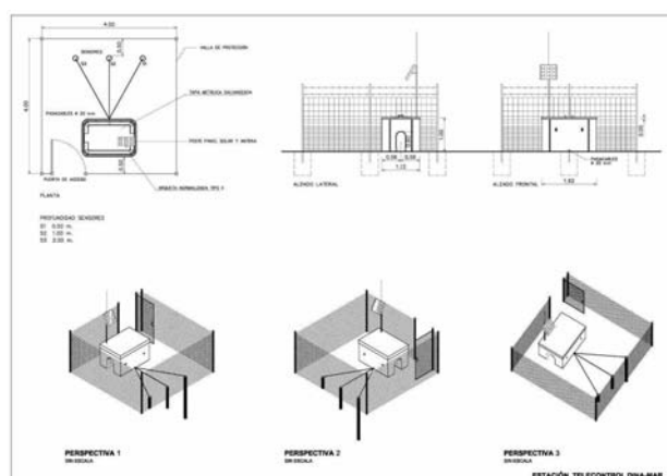
Figura 2. Configuración de las estaciones DINA-MAR ZNS y sensores instalados (tomado de Tragsa, 2008b).
