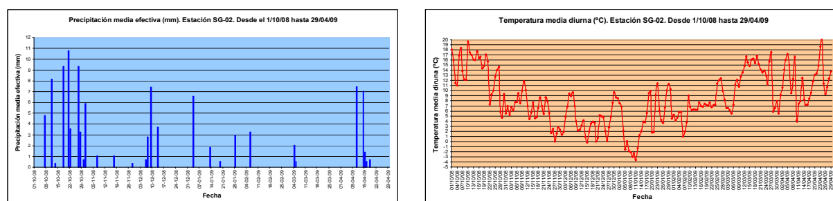
Figura 3 a) y b). Pluviograma y termograma de la estación meteo SG-02, Nava de la Asunción, para la duración del 7º ciclo de gestión de la recarga en la Cubeta de Santiuste.
