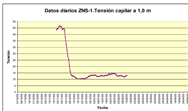
Figura 5. Gráfica de tensión capilar registrada en la estación DINA-MAR ZNS 1. Profundidad del sensor 1,0 m.
