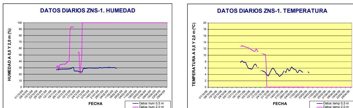
Figuras 4 a) y b). Gráficas de humedad y temperatura registradas en la estación DINA-MAR ZNS 1 de Santiuste para la duración del 7º ciclo de recarga artificial en la Cubeta de Santiuste. Profundidad de los sensores: 0,5 y 2,0 m.
