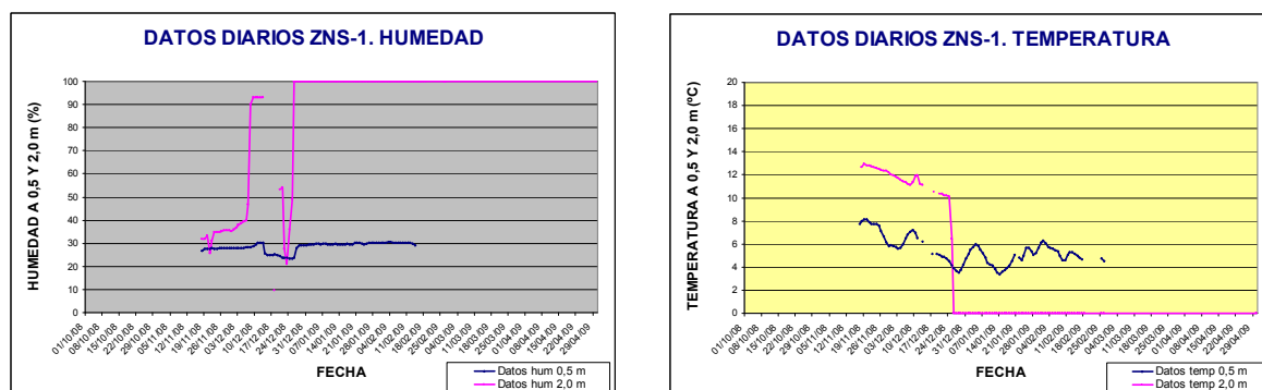
Figuras 4 a) y b). Gráficas de humedad y temperatura registradas en la estación DINA-MAR ZNS 1 de Santiuste para la duración del 7º ciclo de recarga artificial en la Cubeta de Santiuste. Profundidad de los sensores: 0,5 y 2,0 m.
